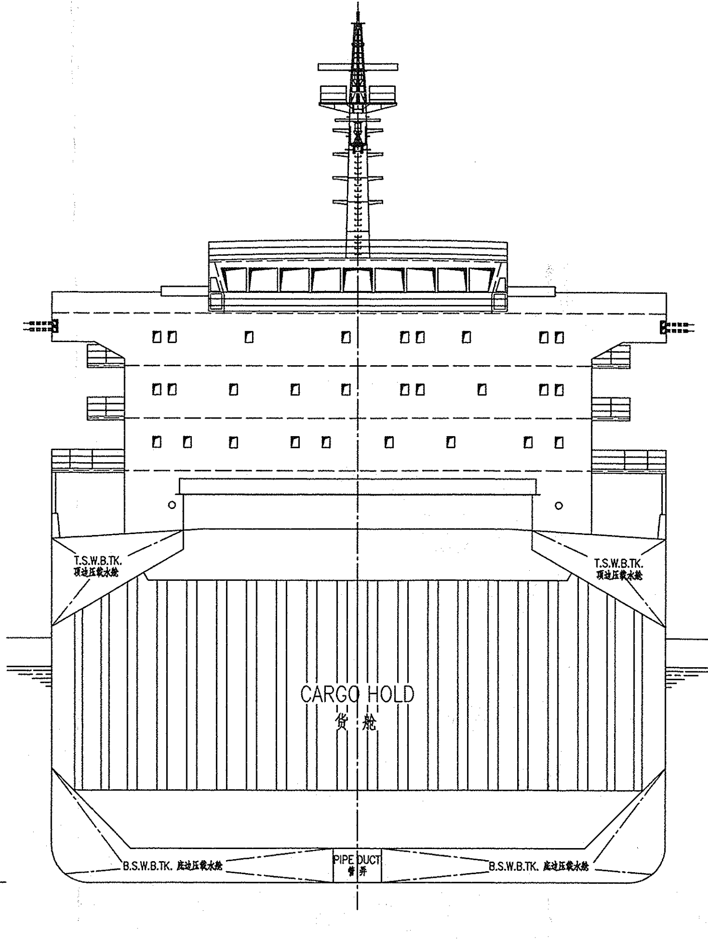
罗经甲板 COMPASS DECK 32100
