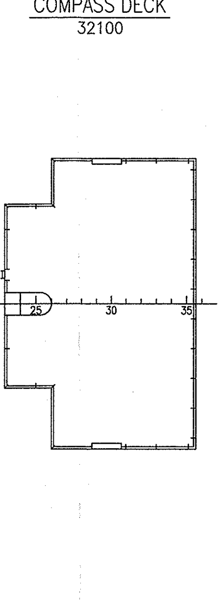
罗经甲板 COMPASS DECK 32100
