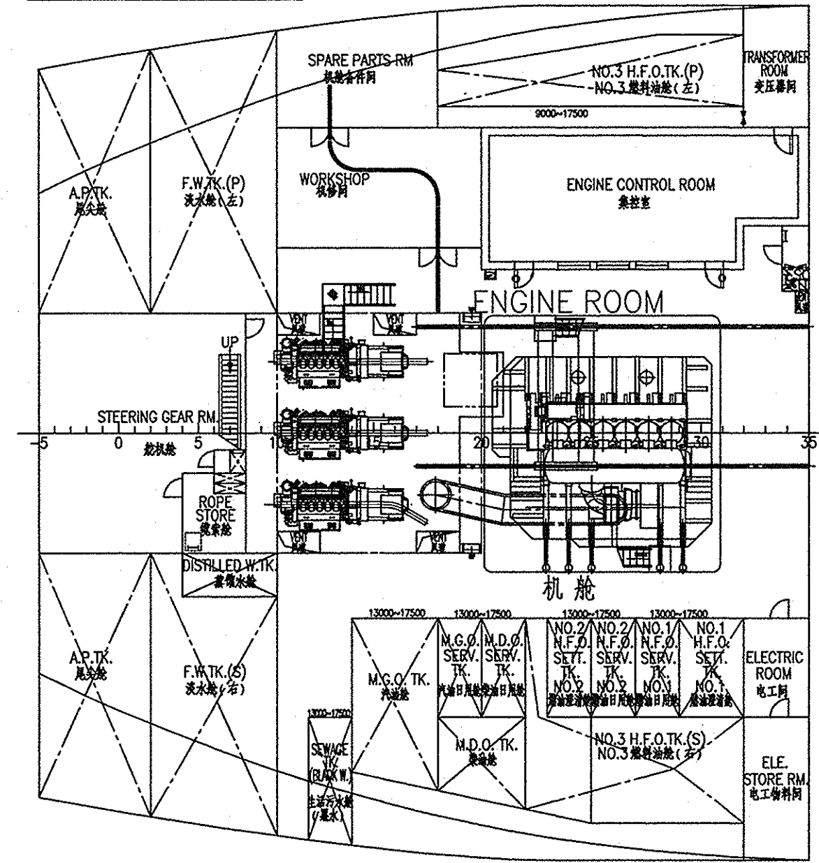
机舱上平台 E/R UPPER PLATFORM
